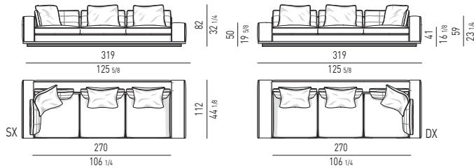
DIVANO ANGOLARE CM 319X112 CORNER SOFA CM 319X112
