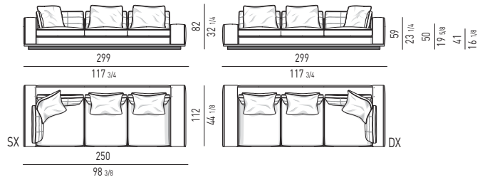
DIVANO ANGOLARE CM 299 CORNER SOFA CM 299
