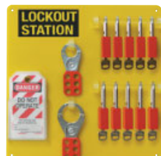
Panneau 10 cadenas Espace pour jusqu'à 12 cadenas
