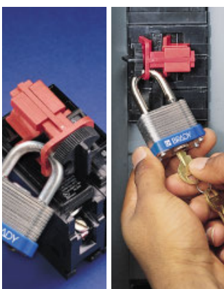
Composants de blocage de disjoncteur - Support de barre de blocage
