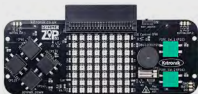
Kitronik :GAME ZIP 64 for the BBC micro:bit SKU: 204-8245 MPN: 5626
