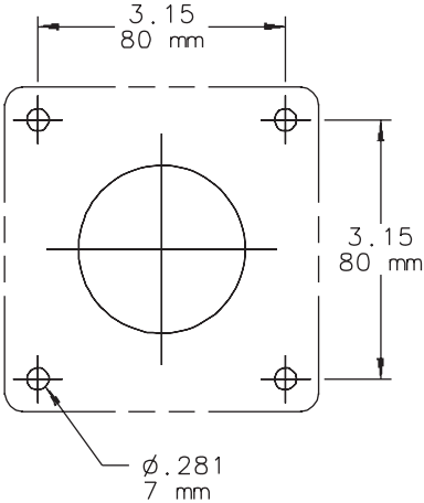
Bottom Pattern diagram du dessous Patrón Inferior
