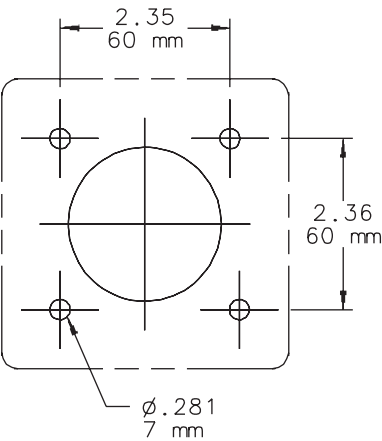
Top Pattern Diagram du dessus Patrón Inferior
