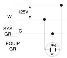
5-15P
