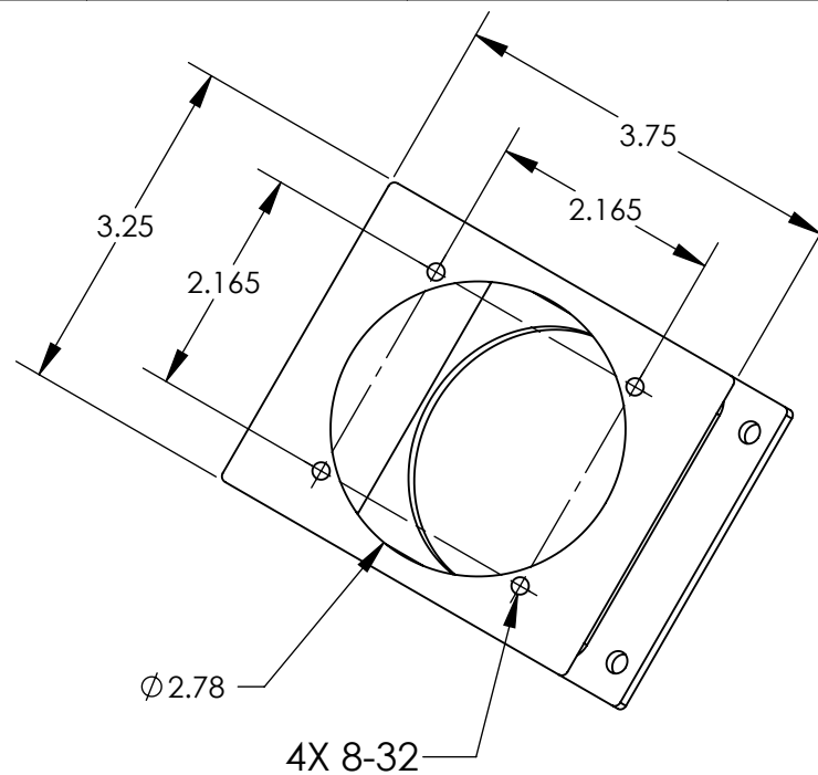
VIEW A-A
