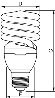
TORNADO T2 23W/850 E26 110-127V 50/60Hz
