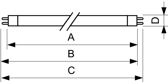
TL5 HO EcoPlus 44=54W/835
