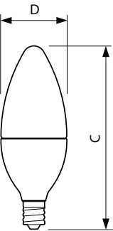
Candle B11 300lm 2700K E12 D CL
