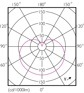
75W E26 A21 FR 250D 822-827 2200-2700K
