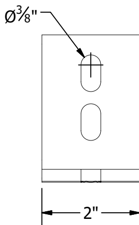
L-FOOT
