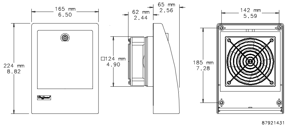
FILTER FAN
