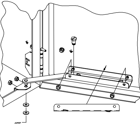
Bottom Mount, Door Right Untere Einfassung, Tür–Recht Bâti Inférieur, Droite De Porte Montaje Inferior, La Derecha De la Puerta
