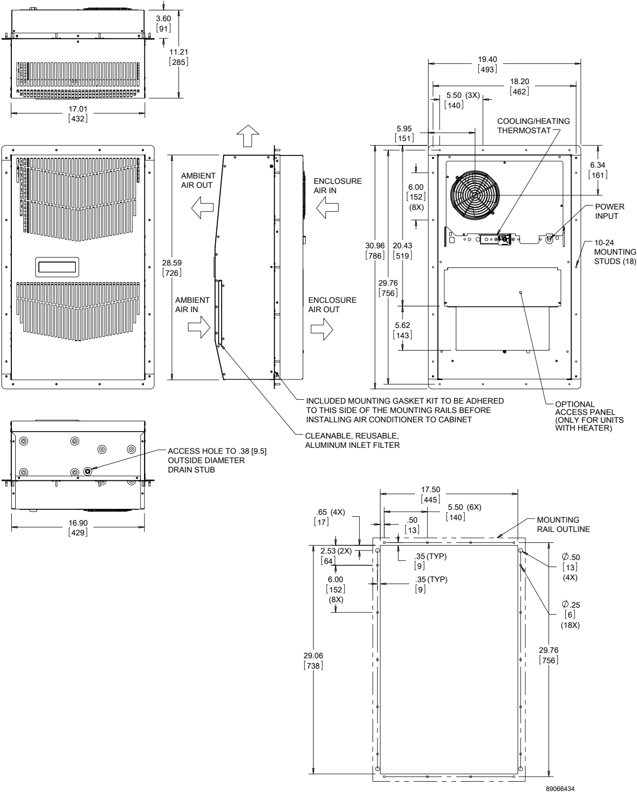
Cutout Dimensions
