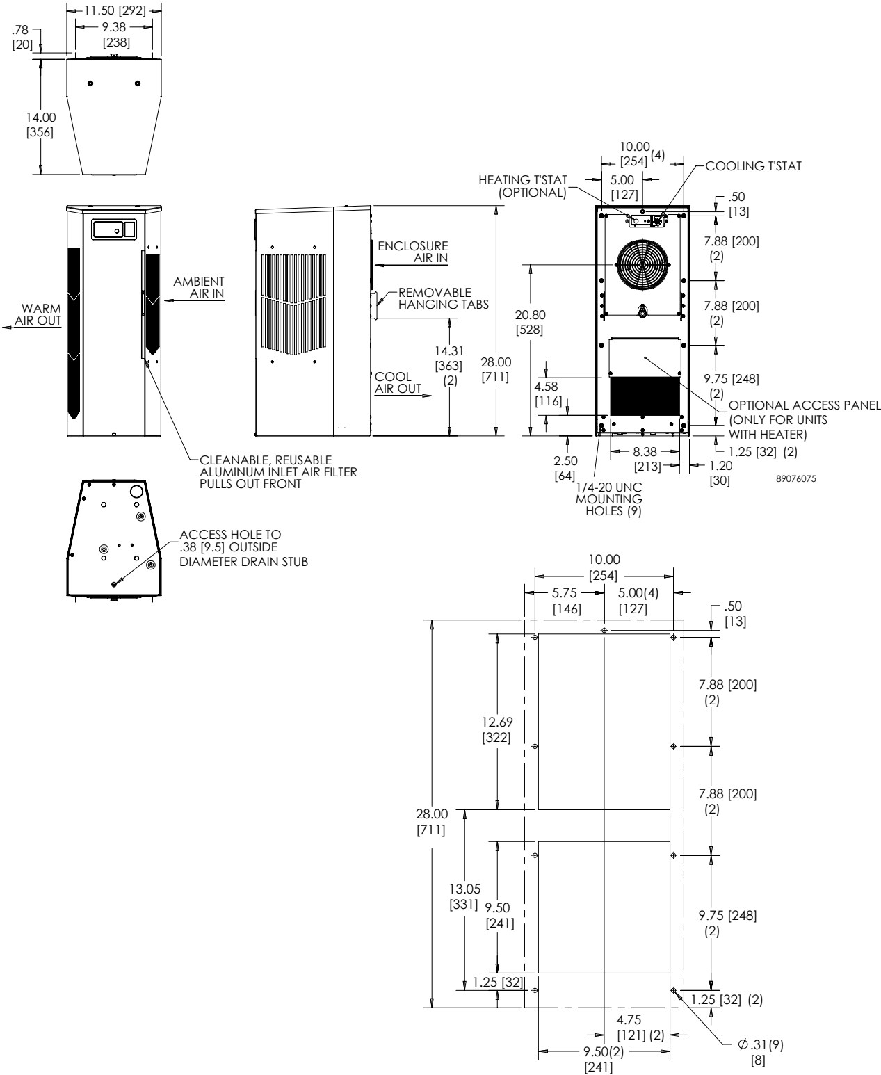
Cutout Dimensions
