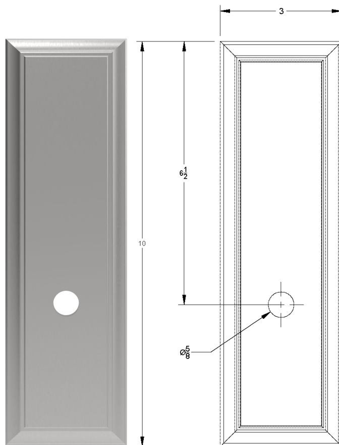
84TE Tubular Escutcheon
