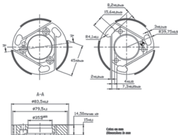
KUPPLUNG MINI
