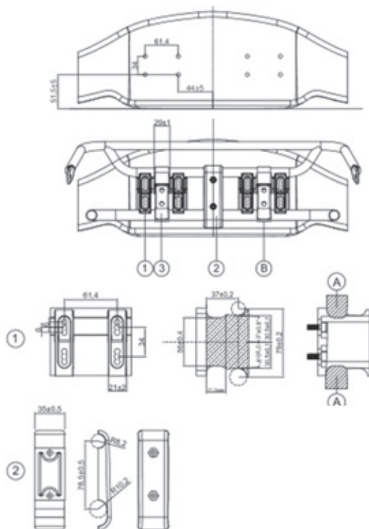
ZEICHNUNG 24 C FRONTVERKLEIDUNGS-BEFESTIGUNGSSATZ MINI
