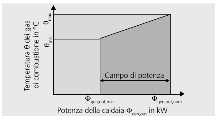
Diagramma della temperatura dei gas combust
