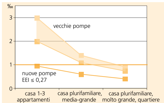
Rapporto tra la potenza elettrica della pompa di circolazione e la potenza termica massima necessaria (potenza termica standard \Phi_{HL} ): regola del per mille, 1‰ = 0,001. Per le zone climatiche più fredde, si avranno dei valori più elevati. Per il riscaldamento a pavimento si avrà un valore maggiorato fino al 50%.
