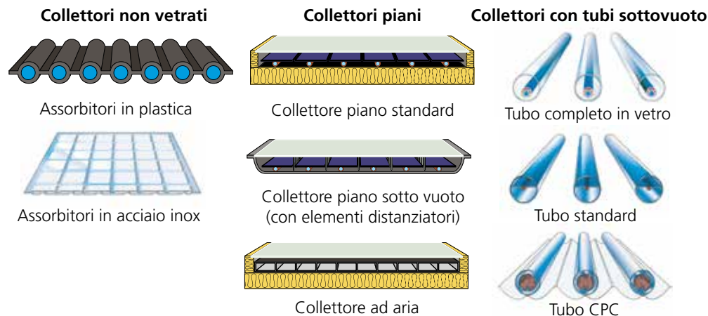
Tipi di collettori solari termici.
