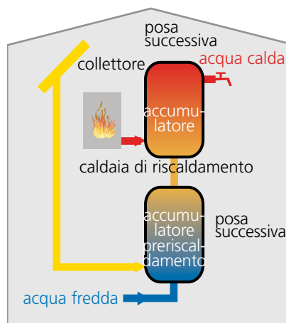
Sistema A: sistema con accumulatore di preriscaldamento 2 accumulatori: accumulatore di preriscaldamento e accumulatore di produzione; semplice ripartizione su diversi accumulatori (spazio); esecuzione successiva semplice.
