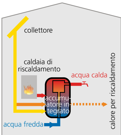
Sistema D: accumulatore combinato. Piccolo accumulatore di produzione integrato nel tampono tecnico; poco fabbisogno di spazio, piccole perdite termiche e brevi tempi di permanenza dell'acqua calda sanitaria; adatto se l'accumulatore esistente dovrà essere sostituito.
