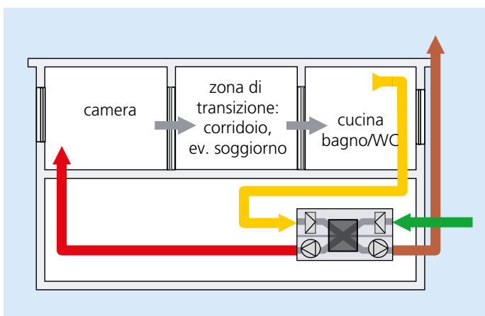
Principio di un'aerazione controllata.
