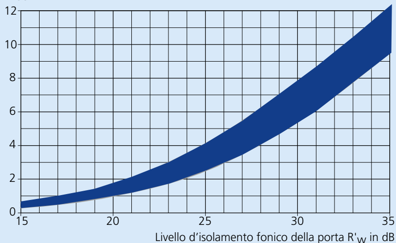
Peggioramento mass. del livello d'isolamento fonico R'_w in dB
