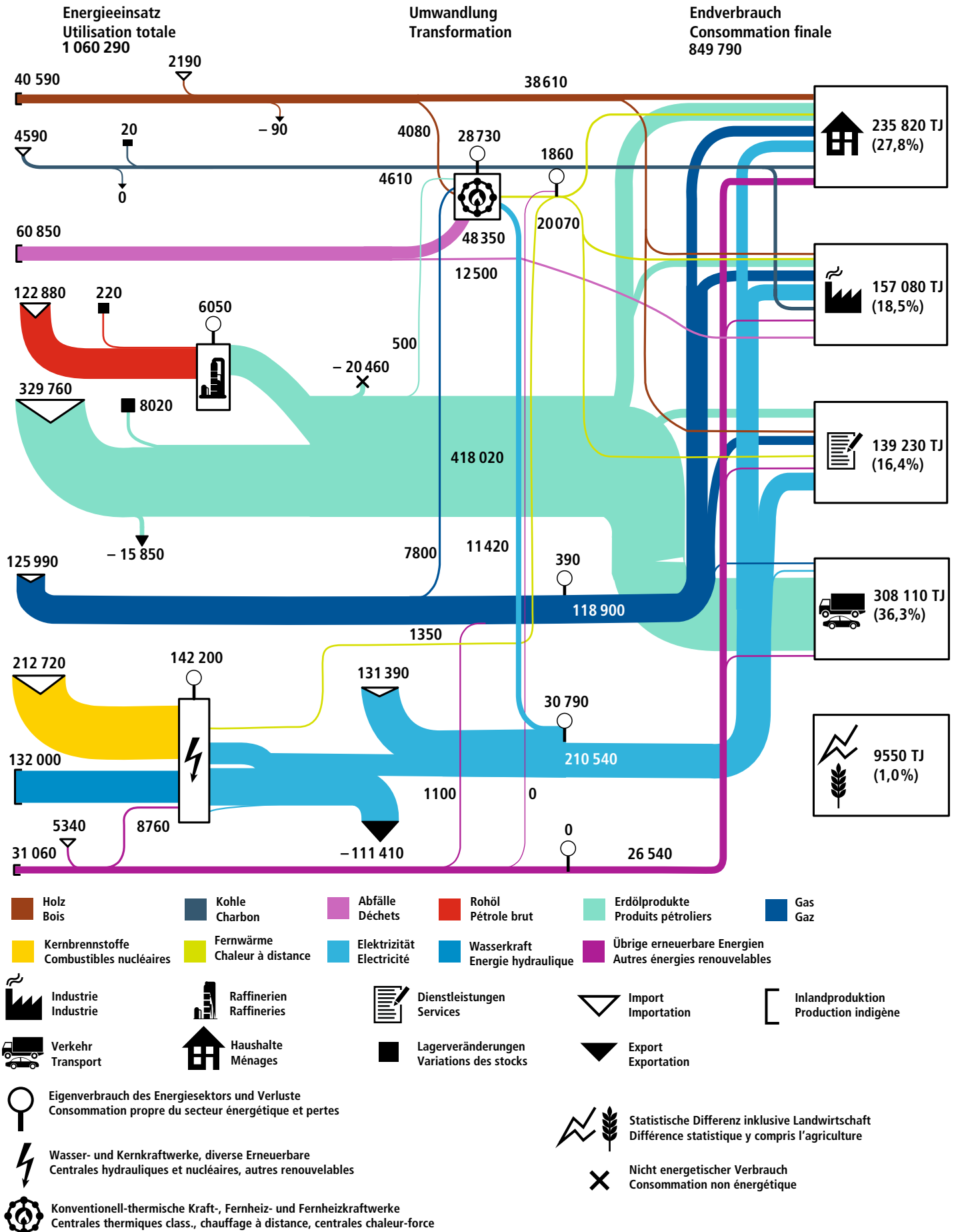
Fig. 5 Detailliertes Energieflussdiagramm der Schweiz 2017 (in TJ) Flux énergétique détaillé de la Suisse en 2017 (en TJ)
