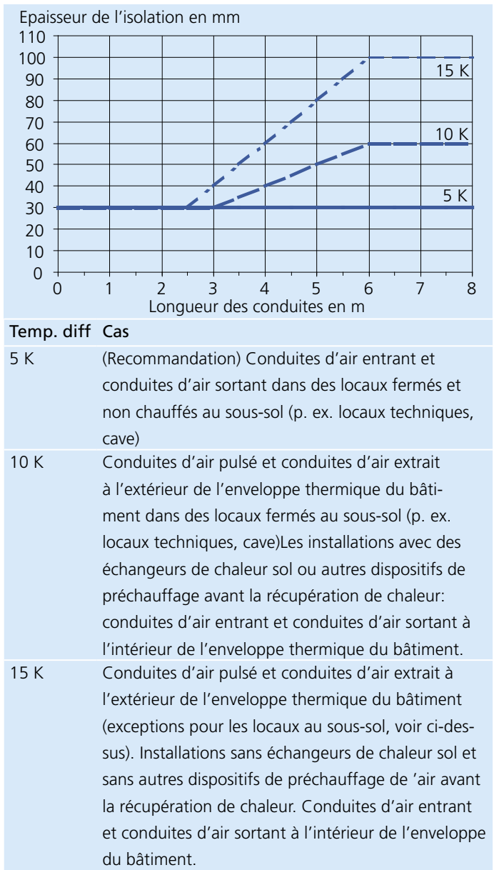
Epaisseur d'isolation minimale de conduites d'air, tuyaux et canalisations en présence d'une isolation thermique présentant une conductivité thermique de 0,03 W/mK <math>\lambda \leq 0,05 \text{ W/mK}</math> [7]
