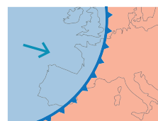
Fronte freddo
