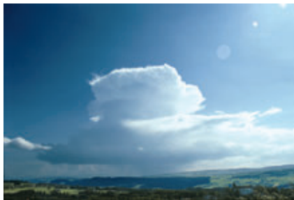
5 Cumulonembo calvo
