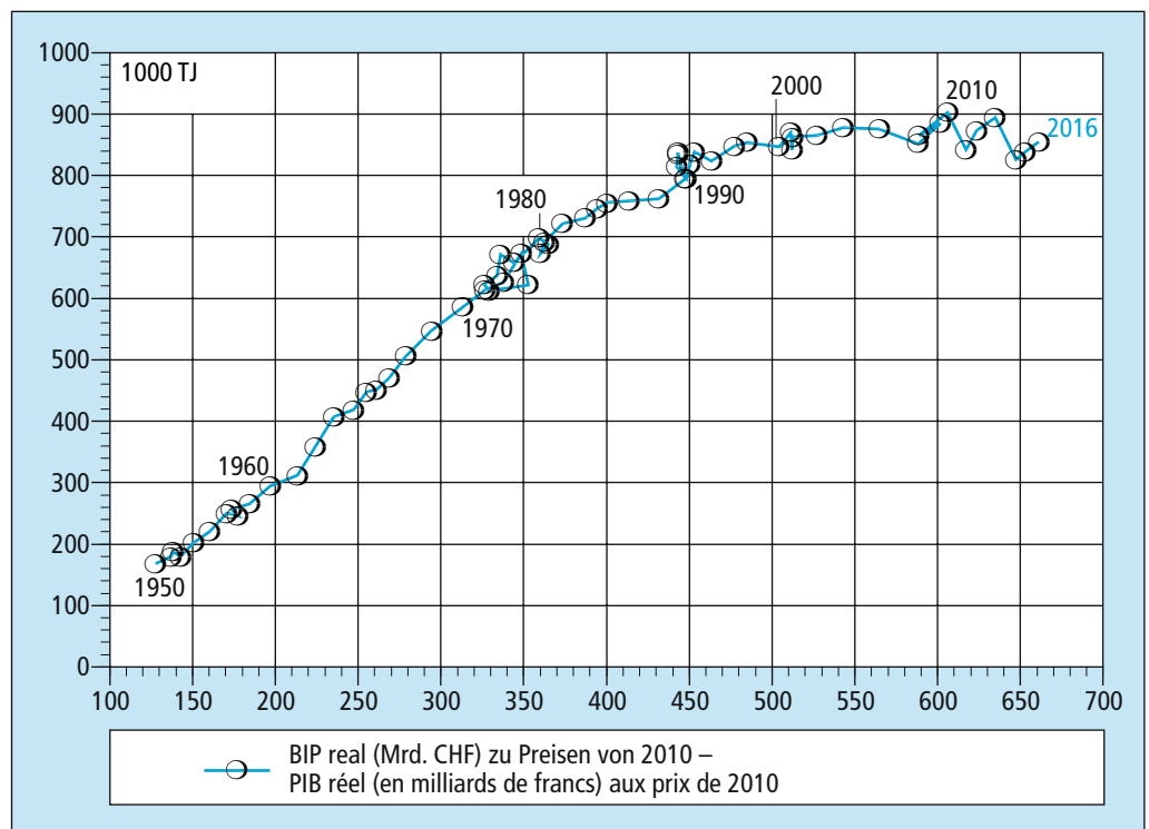
Fig. 15 Zusammenhang zwischen Energieverbrauch und wirtschaftlicher Entwicklung (1950–2016)
