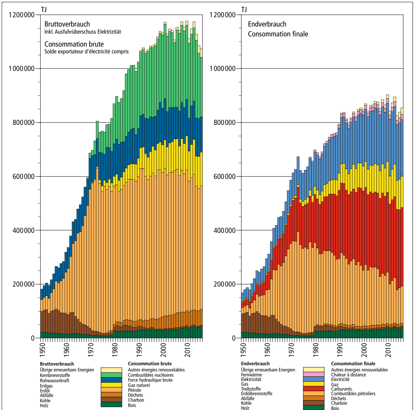
Fig. 4 Energieverbrauch 1950–2016 in Tj Consommation d'énergie 1950–2016 en Tj
