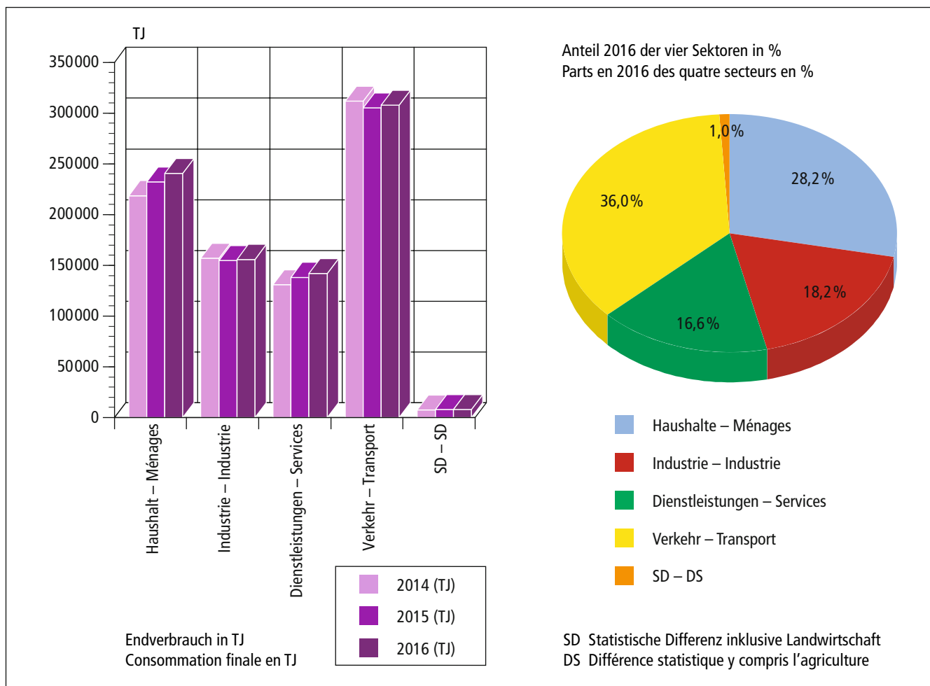
Fig. 3 Aufteilung des Energie-Endverbrauchs nach Verbrauchergruppen (2016) Répartition de la consommation finale d'énergie selon les groupes de consommateurs (2016)
