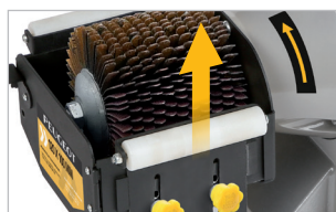
Rouleau d'appui réglable Adjustable tool support
