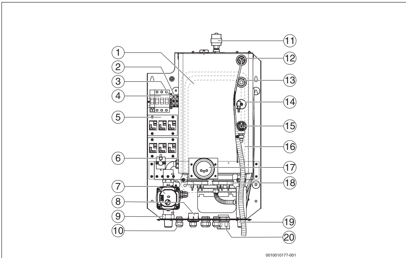
Fig. 2 Éléments de fonctionnement de la chaudière Tronic Heat 3000/Tronic Heat 3500 15-24 kW
