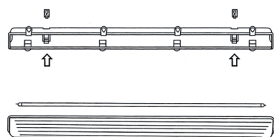
Vue du boîtier ouvert Clips en polycarbonate
