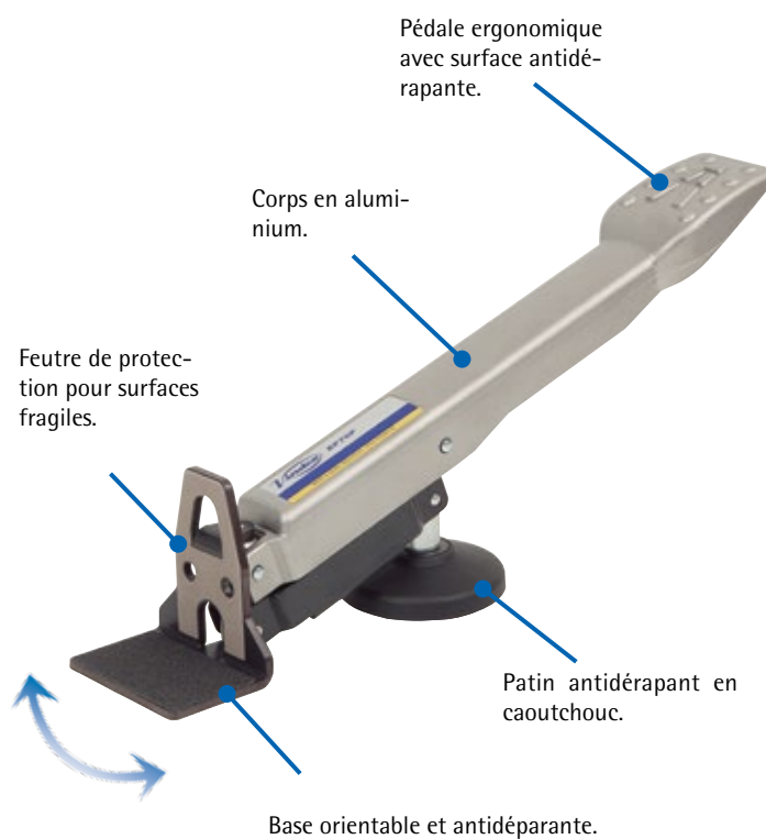
Pour le levage et la mise en place de portes lourdes.
