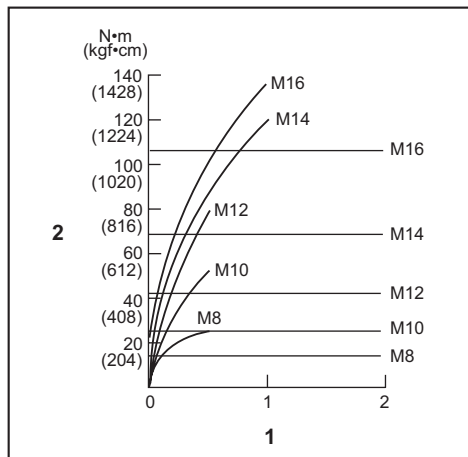
1. Fastspændingstid (sekund) 2. Drejningsmoment
