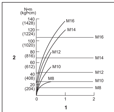
1. Temps de serrage (en secondes) 2. Couple de serrage
