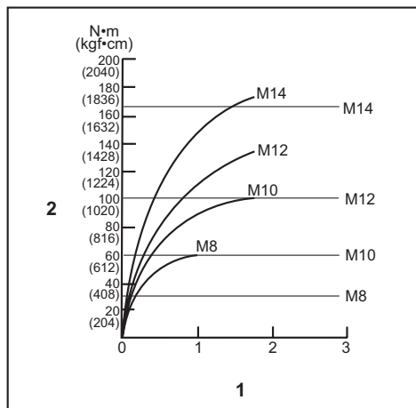
1. Fastspændingstid (sekund) 2. Drejningsmoment
