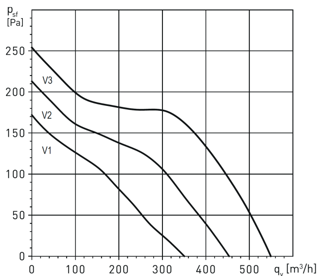
TD 500/150-160 SILENT 3V
