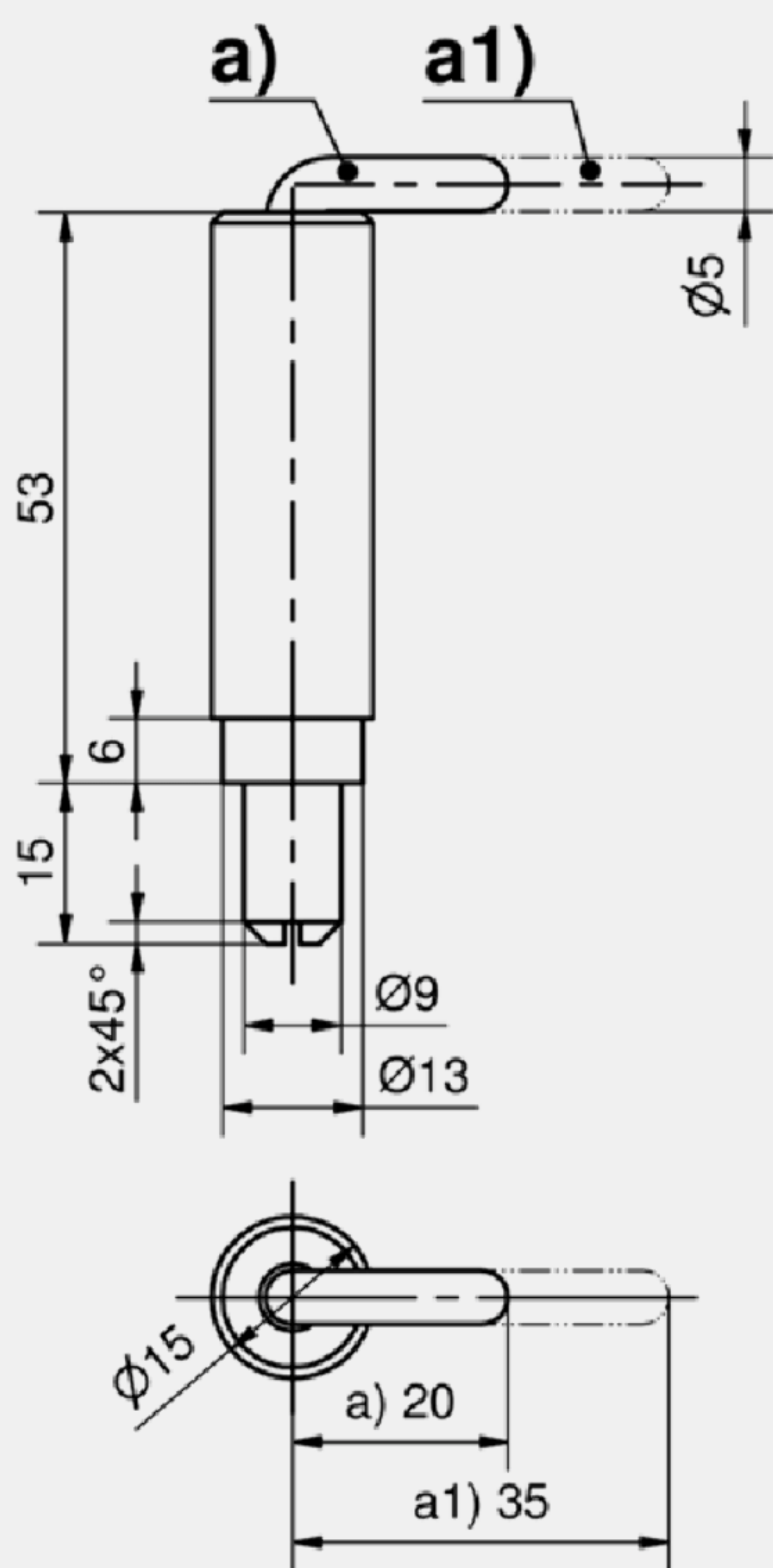
Charnière à broche
