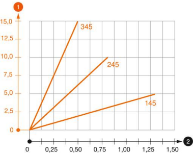
Diagramme de charge du support de plafond TPD
