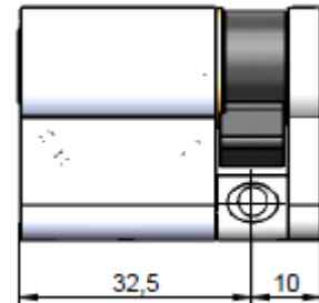
Cylindre simple
