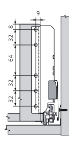
Côtes de montage dos
