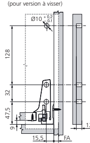
Côtes de montage façade (pour version à visser)
