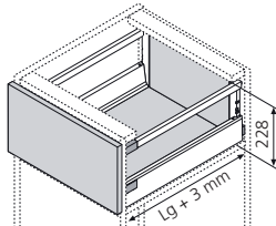
Encombrement
