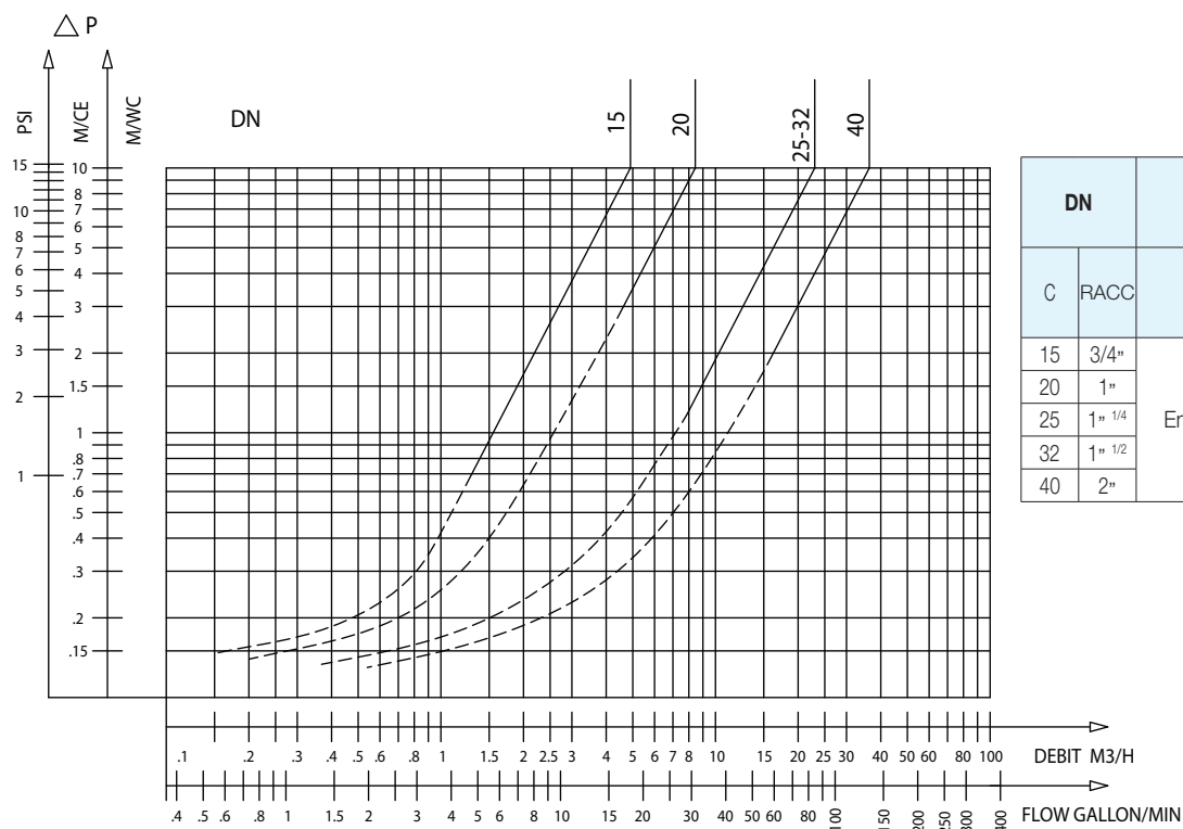
EA 251 - Abaque des pertes de charge
