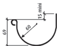
Gouttières demi-rondes de 25
