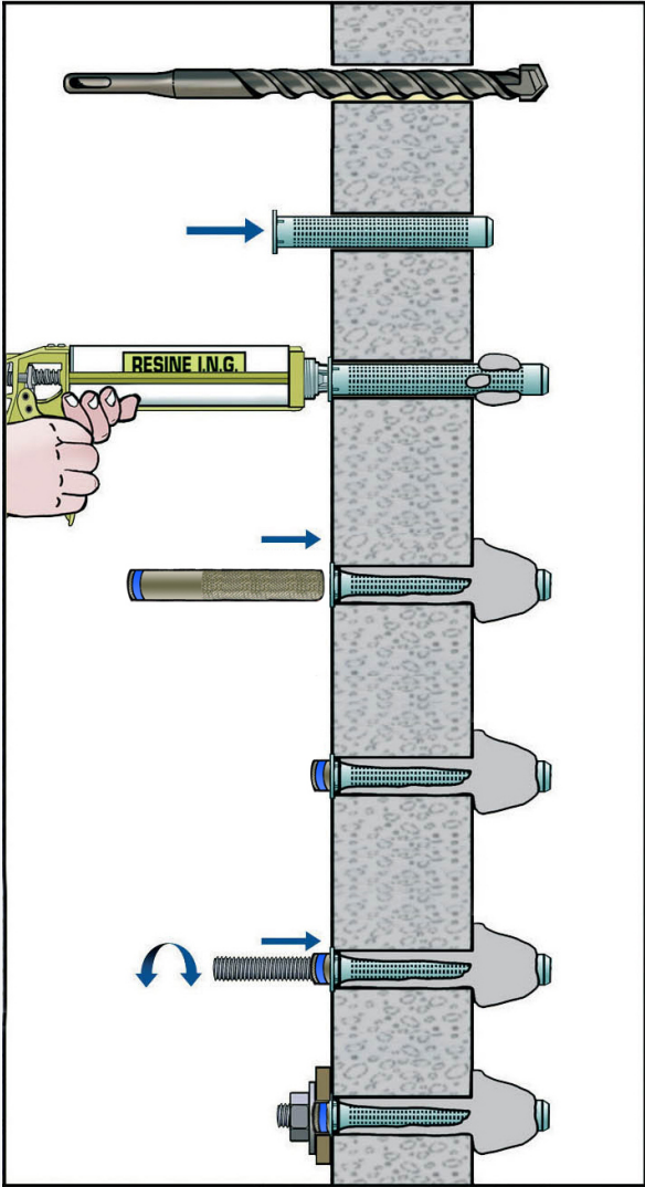
Matériaux creux
