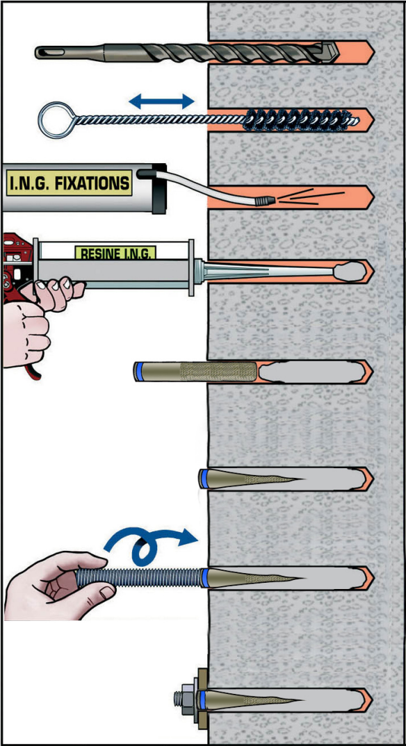
Matériaux pleins
