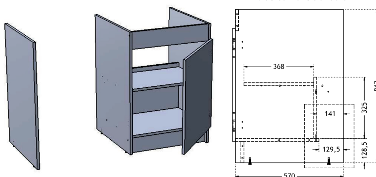
VUE DE DROITE Vide-sanitaire standard
