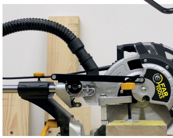
Connexion à un aspirateur Vacuum cleaner connection
