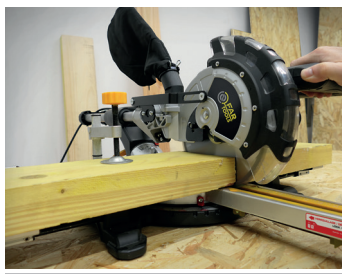
Fonction radiale Radial function
