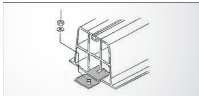
SET DE FIXATION
