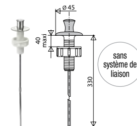
réf. 048100
