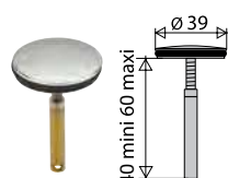
réf. 041200
