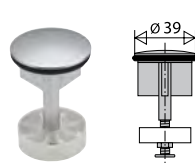
réf. 042800
