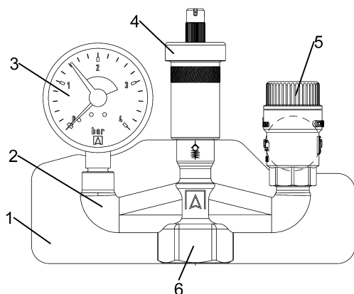
Bild 1: Aufbau der Kesselsicherungsgruppe KSG
