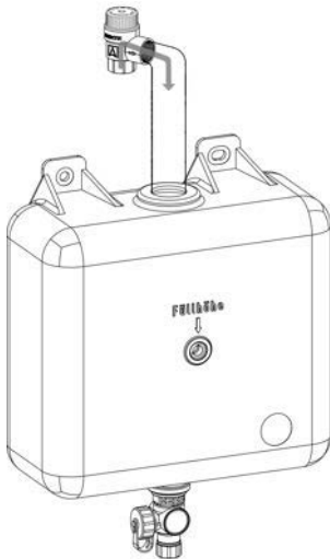
Ilustracja 2: Montaż z przewodem wyrzutowym i zbiornikiem na ciecz solarną
