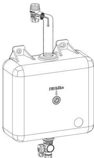
Figura 2: Montare cu conductă de evacuare și container de colectare specific pentru instalații solare
