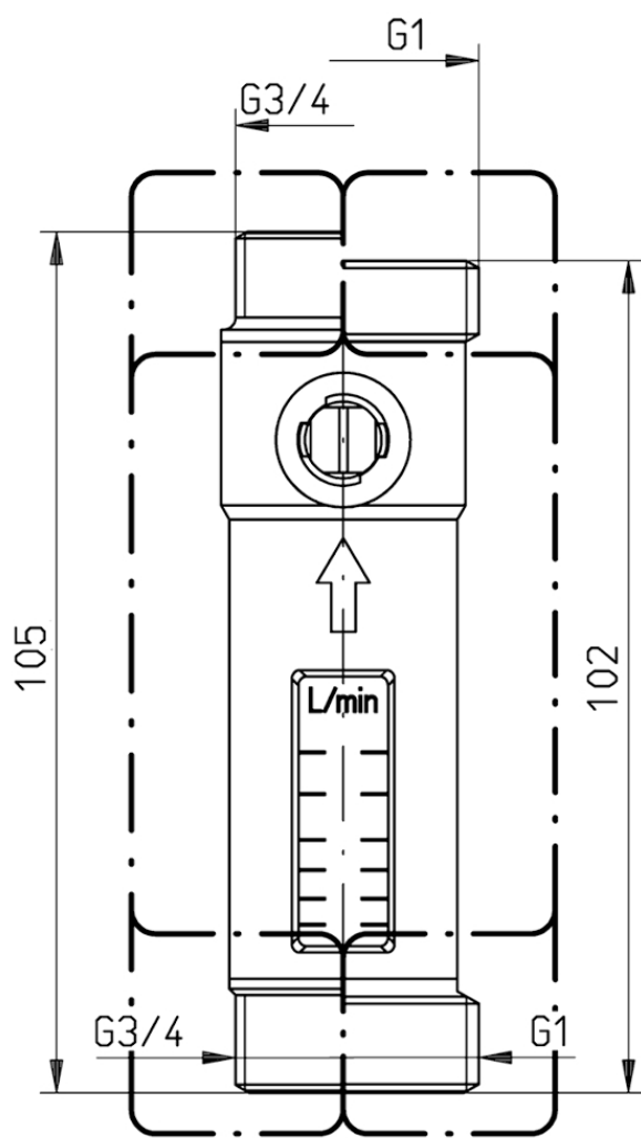
DFM 15-2M, Aussengewinde x Aussengewinde
