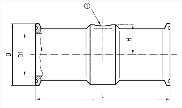
Type RD 60 Clamp ISO 2852
