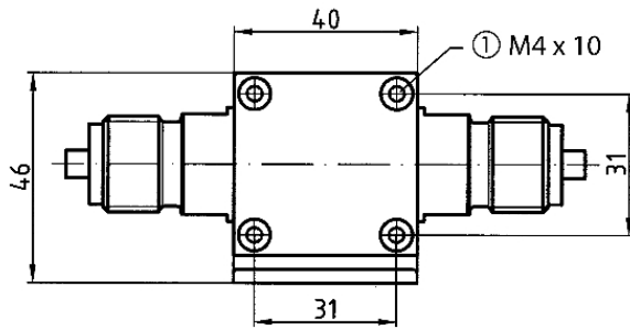
DMU 11 D - connection 2 x G \frac{1}{2} B (EN 837)
