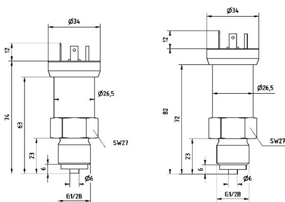
DMU 05 P - connection G \frac{1}{2} B EN 837
