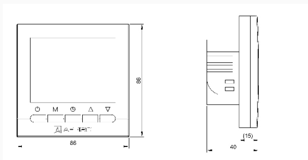
Masse (mm)
