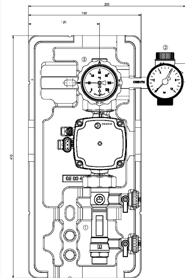
solar pump line PrimoSol® 130-1
