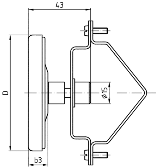
Anschluss axial, mit Universalschelle für Rohre 3/4" bis 1 1/2"
