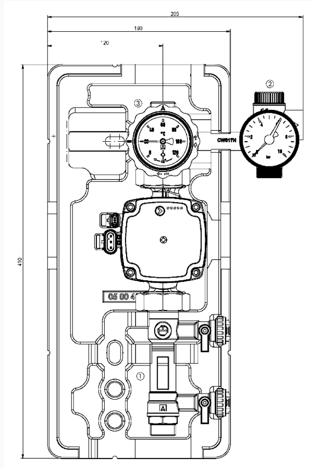
solar pump line PrimoSol® 130-1
