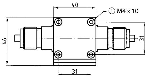
DMU 11 D - connection 2 x G½B (EN 837)
